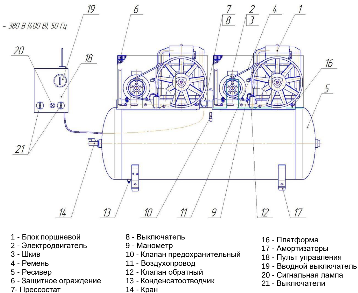
Рисунок 4 - Общий вид компрессора СБ4/Φ-500.AB998ТБ
